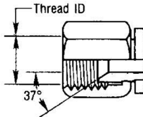
JIC 37° Flare
